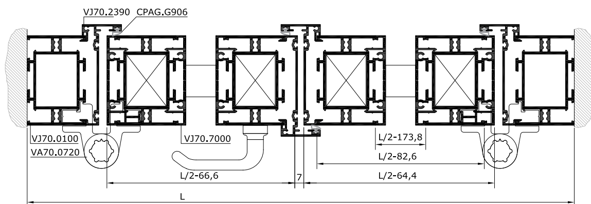
SECCIÓN HORIZONTAL
