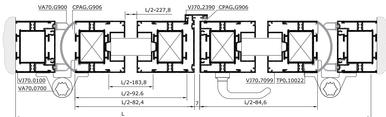
SECCIÓN HORIZONTAL
