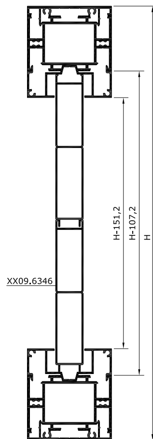
SECCIÓN VERTICAL
