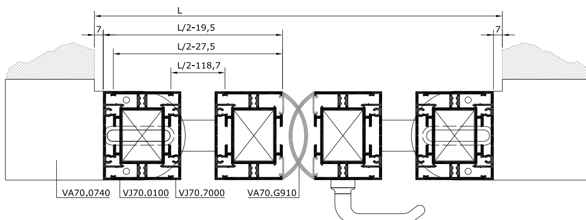
SECCIÓN HORIZONTAL
