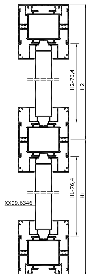
SECCIÓN VERTICAL
