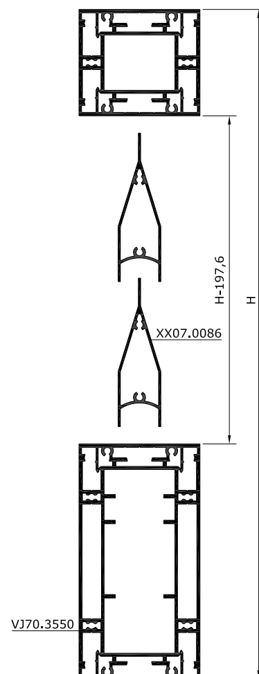
SECCIÓN VERTICAL
