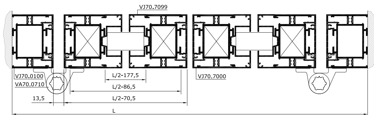
SECCIÓN HORIZONTAL
