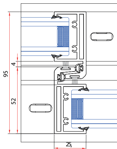
SECCIÓN HORIZONTAL CRUCE
