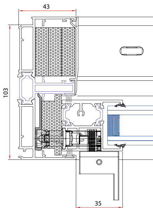
SECCIÓN HORIZONTAL
