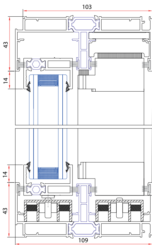
SECCIÓN VERTICAL
