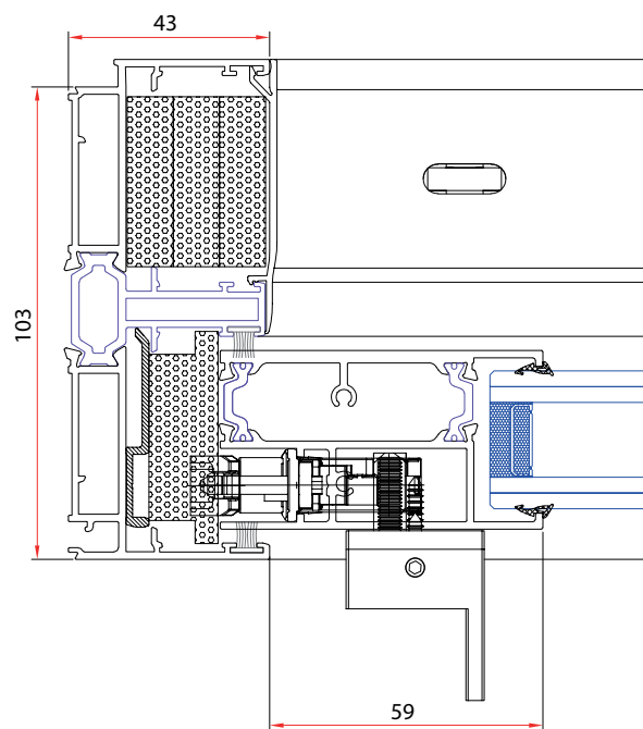
SECCIÓN HORIZONTAL SEGURIDAD
