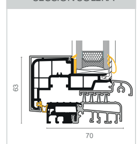
SECCION SOLERA
