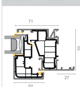
SECCION MARCO SOLAPE
