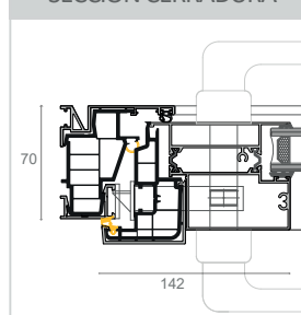
SECCION CERRADURA
