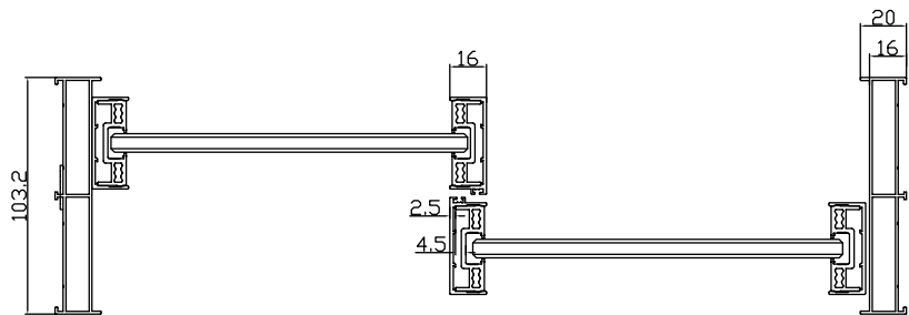
SECCION : A-A
