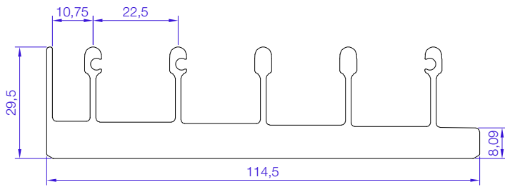
MARCO INFERIOR 5 CARRILES
