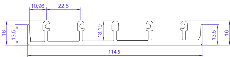
MARCO INFERIOR EMPOTRADO 5 CARRILES
