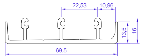
MARCO INFERIOR EMPOTRADO 5 CARRILES
