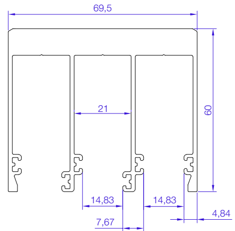
MARCO INFERIOR 3 CARRILES
