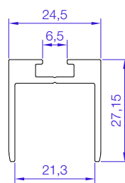
PERFI COMPENSADOR MARCO LATERAL
