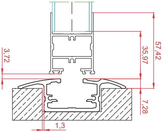
GUÍA INFERIOR EMPOTRADA Y HOJA HORIZONTAL
