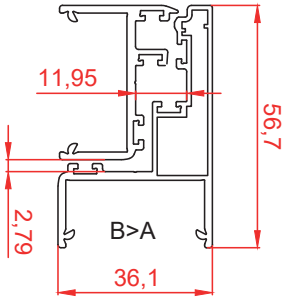
HOJA VERTICAL CON HOJA VERTICAL ESQUINA 90°
