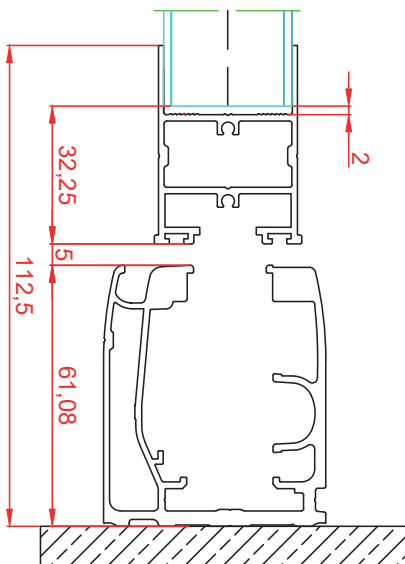
GUÍA INFERIOR Y HOJA HORIZONTAL
