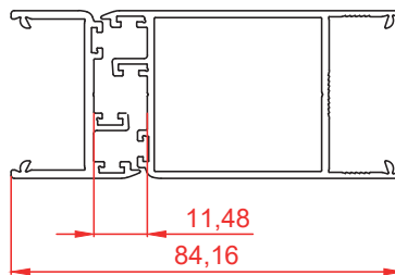
HOJA VERTICAL CON ESPAÑOLETA
