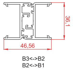
HOJA VERTICAL CON HOJA VERTICAL
