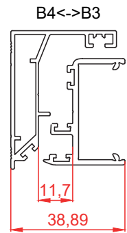
HOJA VERTICAL CON MARCO LATERAL
