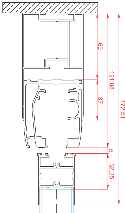
PERFIL DE COMPENSACIÓN, GUÍA SUPERIOR Y HOJA HORIZONTAL
