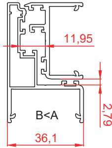
HOJA VERTICAL CON HOJA VERTICAL ESQUINA 90°
