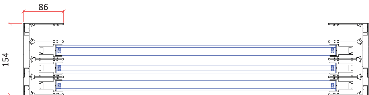
SECCIÓN HORIZONTAL DE ZENLINE VERTICAL UP 3 HOJAS
