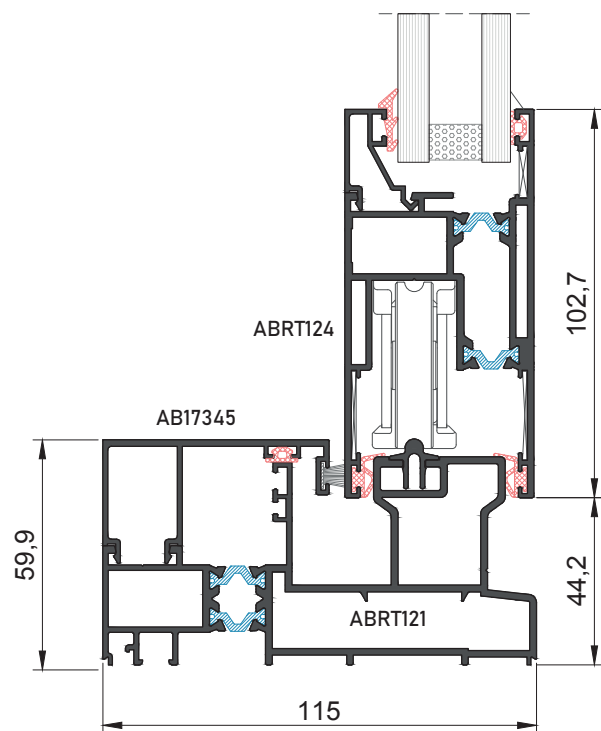
Sección 7
