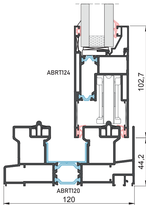
Sección 2
