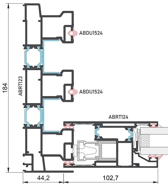
Sección 1
