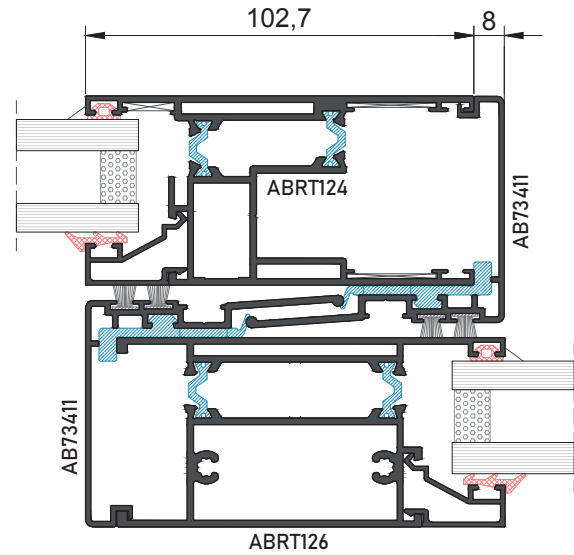
Sección 2
