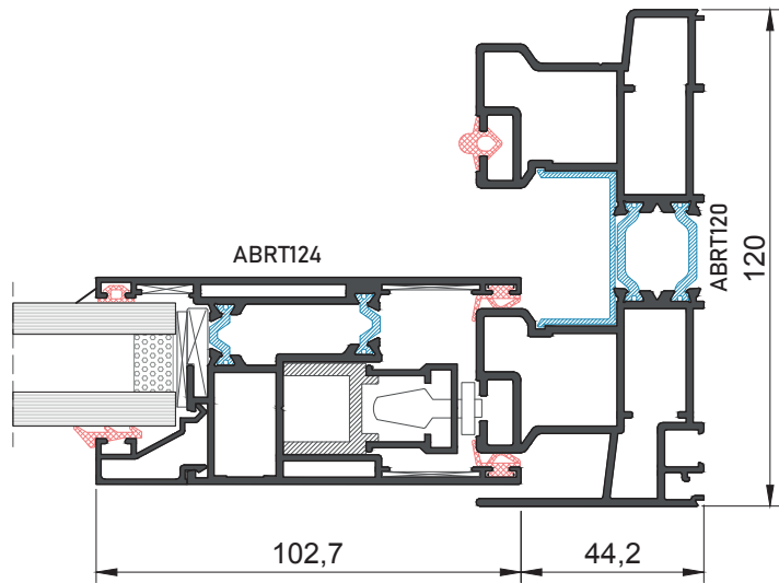
Sección 4
