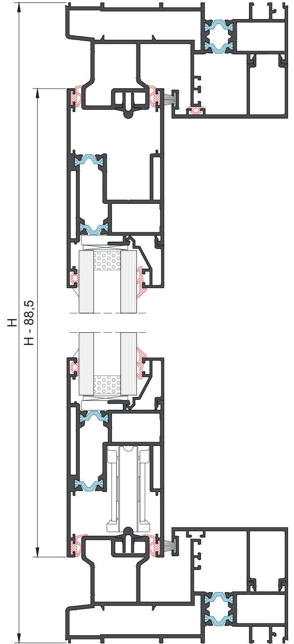
SECCIÓN VERTICAL
