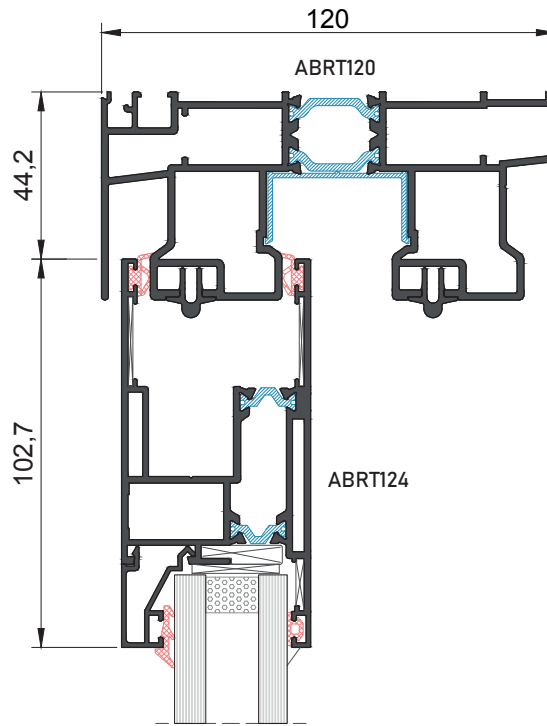
Sección 1
