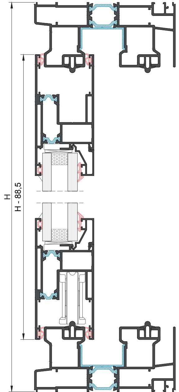
SECCIÓN VERTICAL
