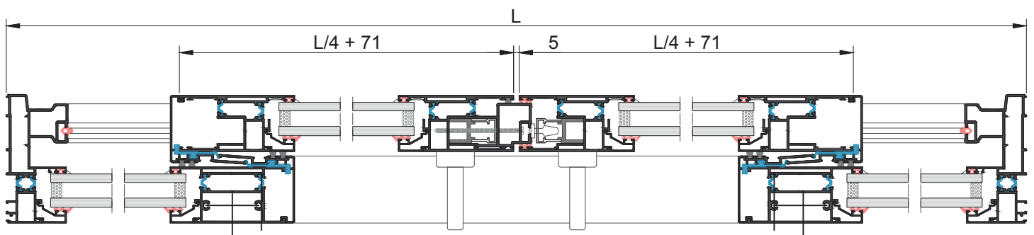
SECCIÓN HORIZONTAL
