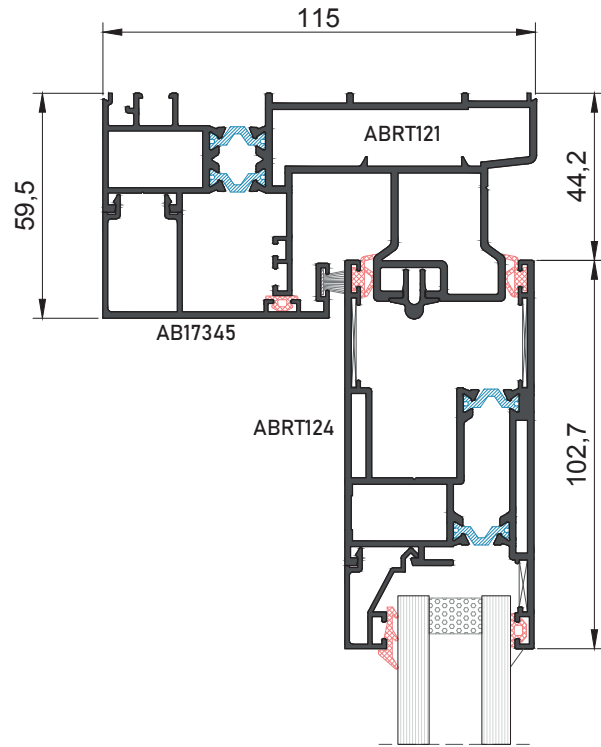
Sección 6
