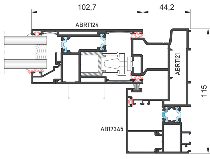
Sección 3
