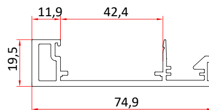
HOJA CRUCE FIJOS 40
