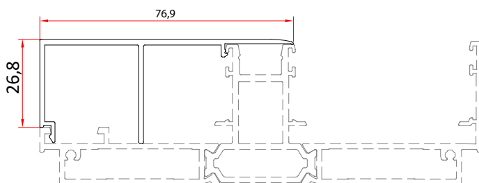
TAPA MARCO FIJO
