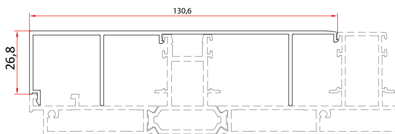
TAPA FIJO TRICARRIL
