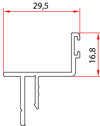
PERFIL LATERAL MARCO
