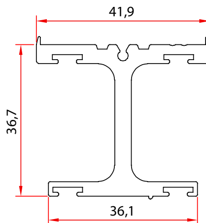
GUÍA INFERIOR
