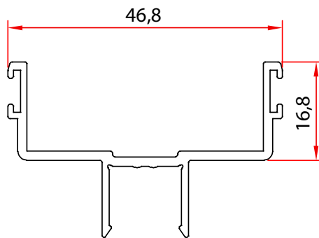
GUÍA INFERIOR
