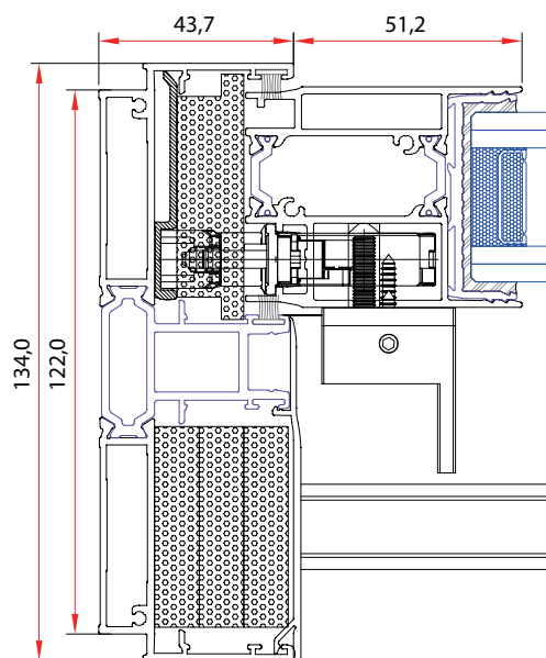
SECCIÓN HORIZONTAL SEGURIDAD
