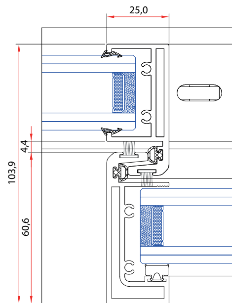
SECCIÓN HORIZONTAL CENTRAL
