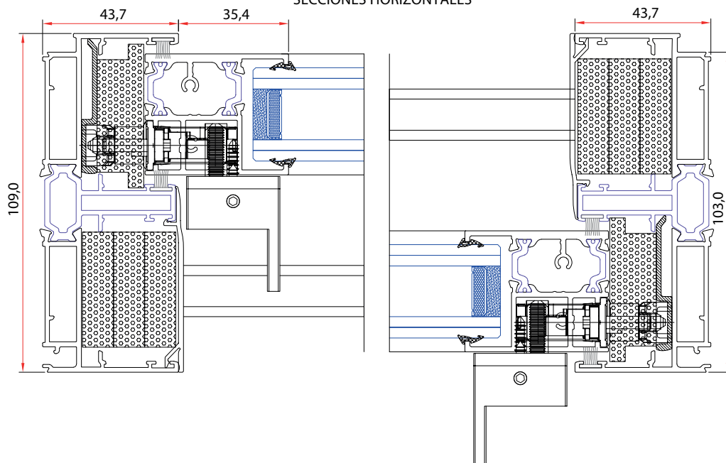
SECCIONES HORIZONTALES
