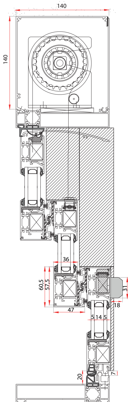
SECCIÓN VERTICAL 3 HOJAS
