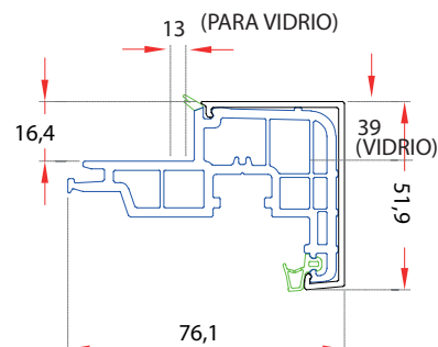
HOJA
