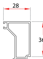
JUNQUILLO MARCO
