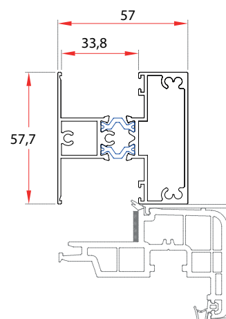
TRAVESAÑO HOJA
