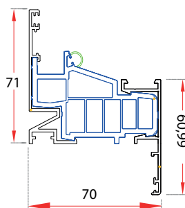
MARCO SOLAPE
