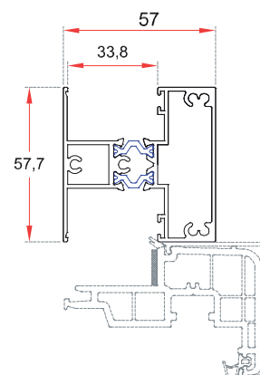
TRAVESAÑO HOJA
