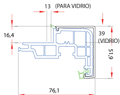
HOJA
