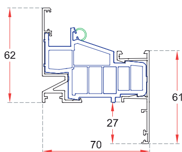
MARCO SOLAPE
