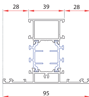
TRAVESAÑO MARCO
