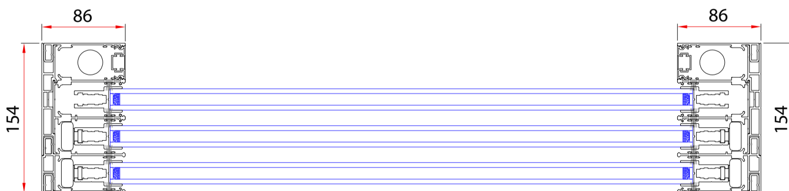
Sección Horizontal de Zenline Vertical Up 3 hojas
