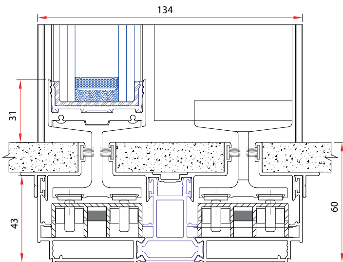
SECCIÓN HORIZONTAL CENTRAL
