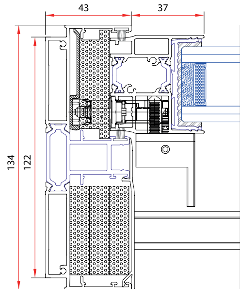
SECCIÓN HORIZONTAL
