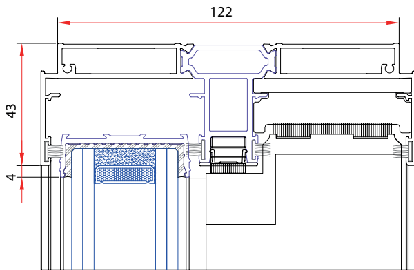
SECCIÓN VERTICAL
