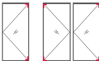
BISAGRAS PUNTO DE GIRO (180°)
