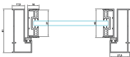
SECCION 1 HOJA
