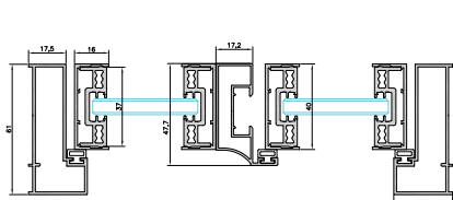
SECCIONES 2 HOJAS
