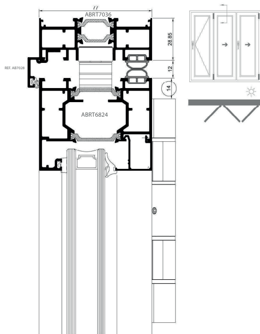
Detalle sección superior Detalle colocación bisagra patín superior
