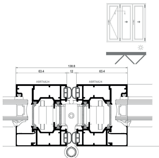
Detalle sección horizontal encuentro hojas con patín
