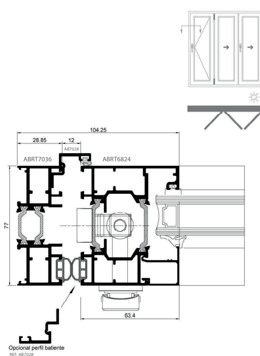
Detalle sección horizontal hoja batiente
