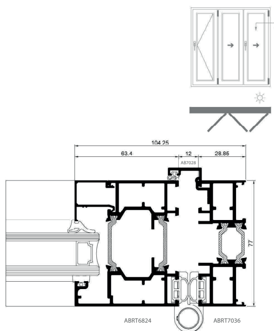
Detalle sección horizontal hoja batiente
