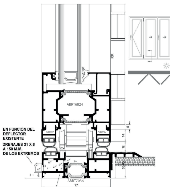
Detalle drenaje marco inferior DE 10 X 4 M.M. CENTRADO POR CADA HOJA
