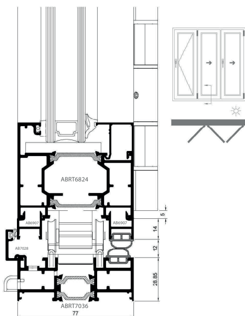
Detalle colocación bisagra patín inferior
