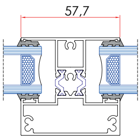
Sección Vertical Travesaño Hoja
