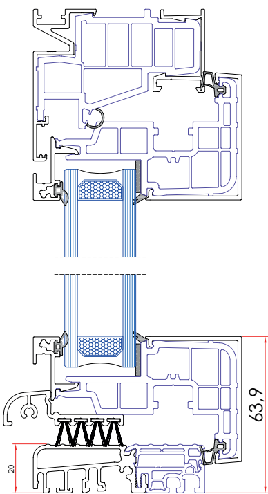
Sección Vertical con Solera
