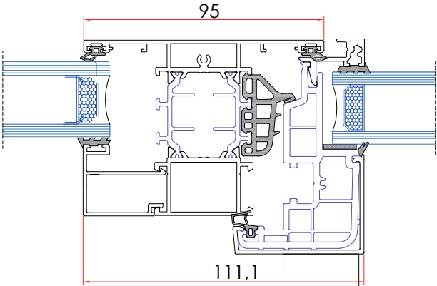
Sección Horizontal Travesaño Marco
